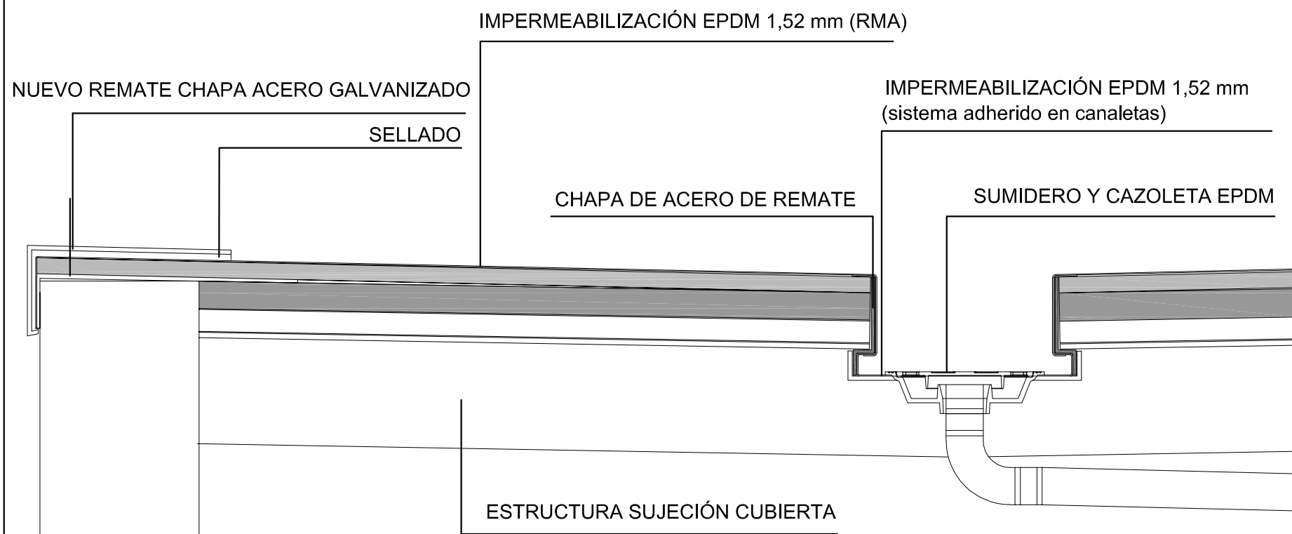
SECCIÓN ESTADO REFORMADO
