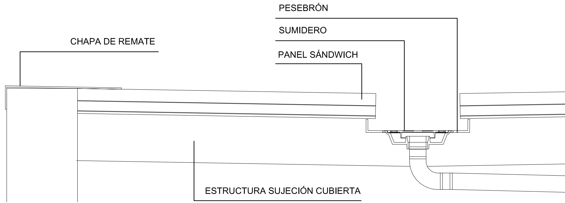
SECCIÓN ESTADO ACTUAL
