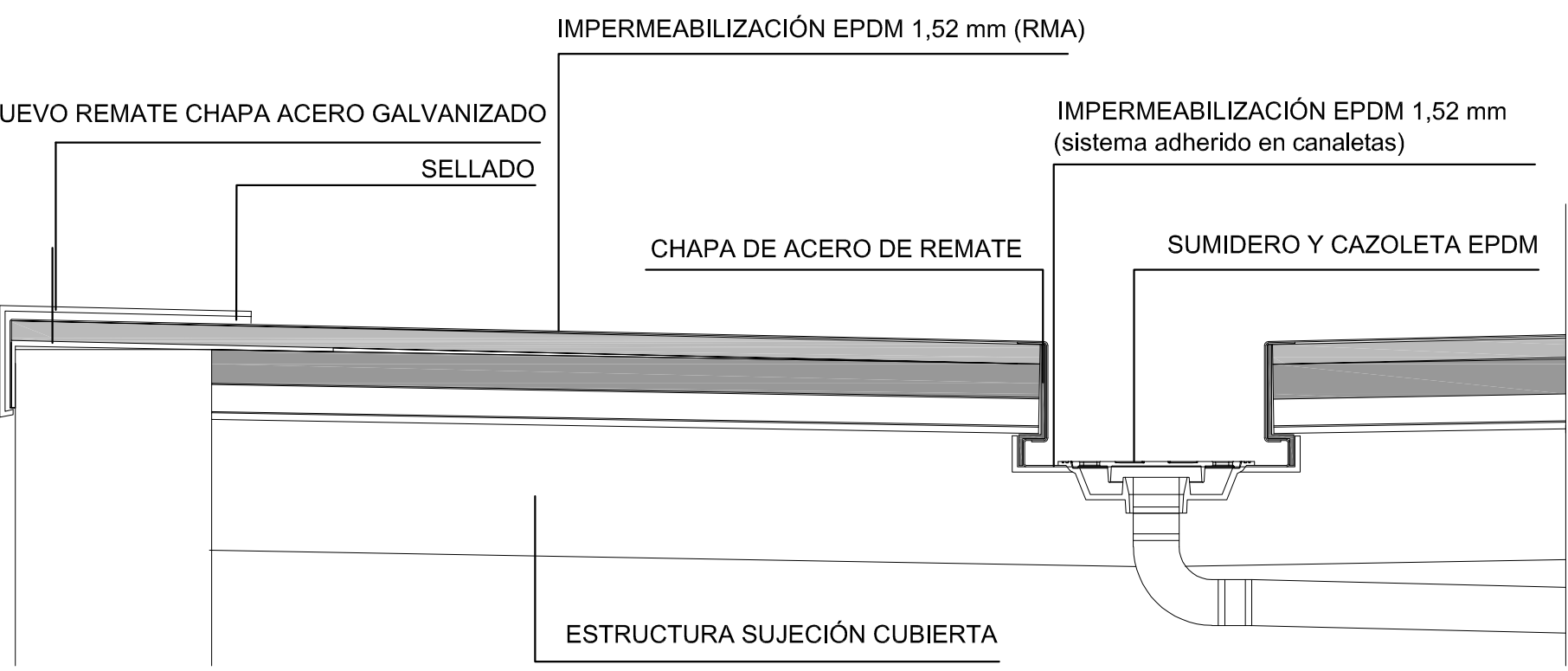
SECCIÓN ESTADO REFORMADO
