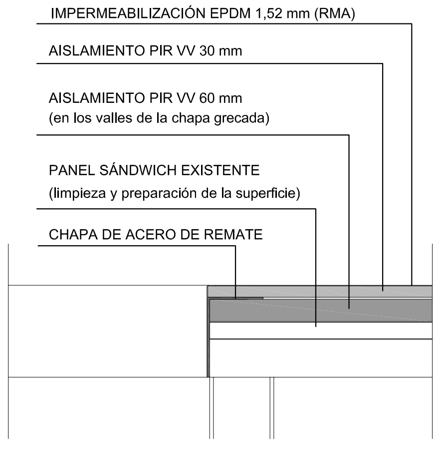
SECCIÓN ESTADO REFORMADO
