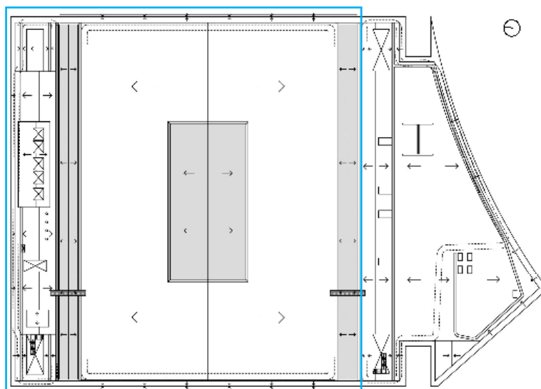
Planta general de cubierta, zonas de intervención
