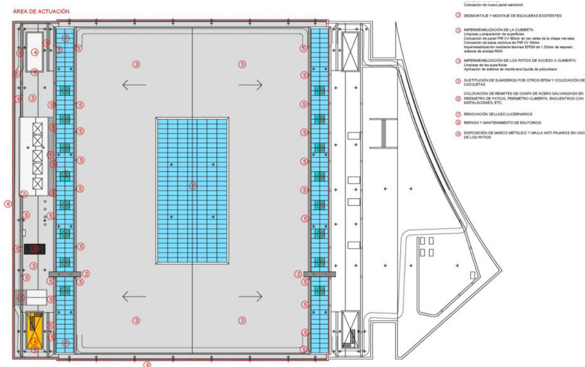
Actuaciones en planta de cubiertas
